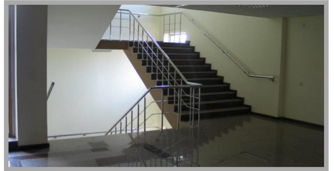
İç mekan merdiven 3 emniyet kayıtlı üstten bağlantılı korkuluk uygulaması
